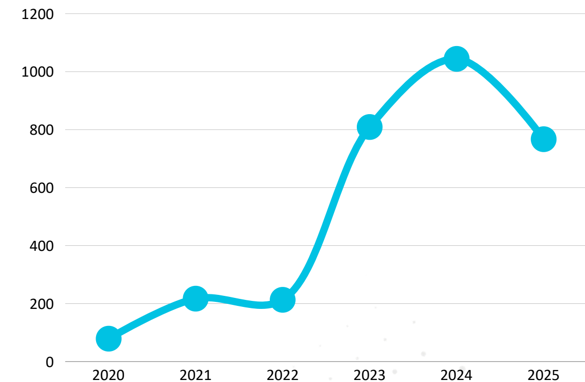
Évolution du nombre de trajets en covoiturage par an
