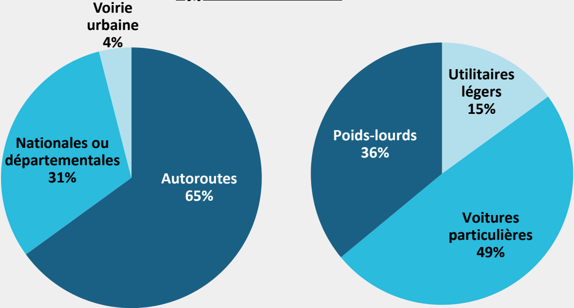
Émission de GES, par type de route et par type de véhicule
