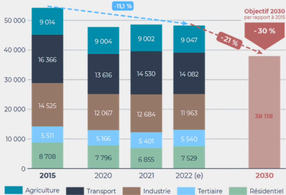
Trajectoire territoriale des émissions de gaz à effet de serre
